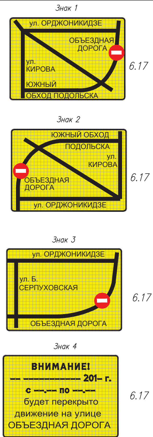
Ведомость дорожных знаков
